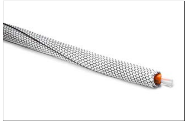
Funda auto-cerrable repelente a roedores en aplicación en cable de fibra óptica.
